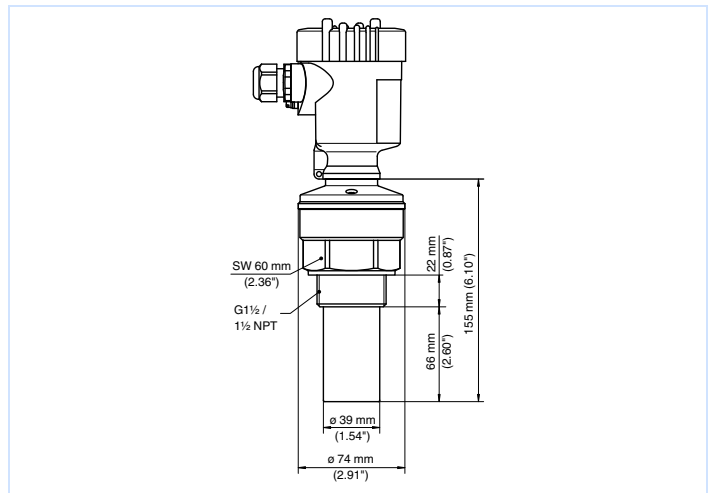
Размеры VEGASON 61
