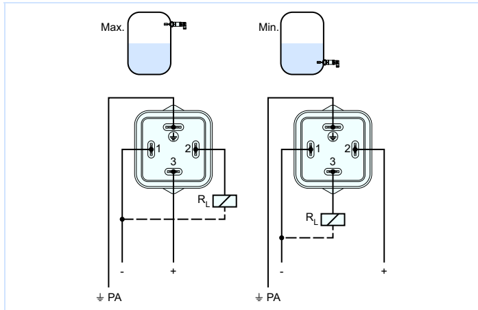
VEGASWING 51 со штекером по ISO 4400
