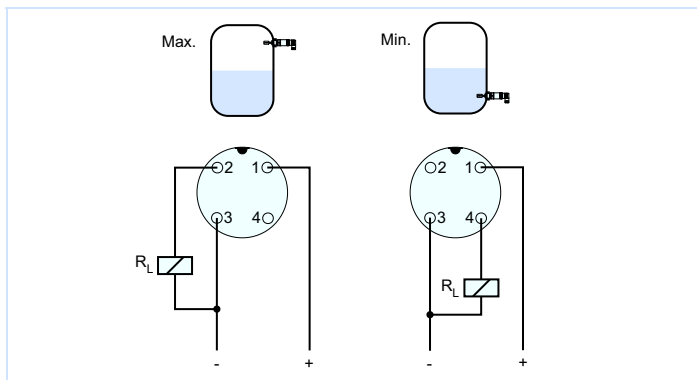
VEGASWING 51 с штекерным разъемом M12 x 1
