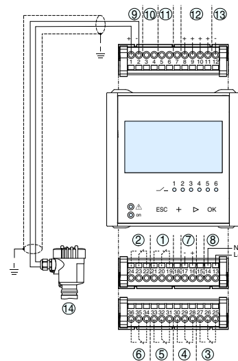
Подключение VEGAMET 391 и двухпроводного датчика
