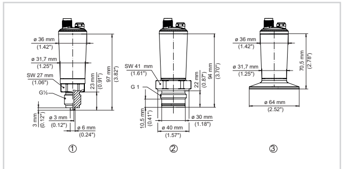
Размеры VEGABAR 29
