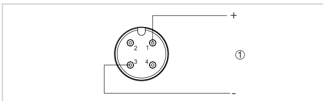
Схема подключения - 2-провод. 4 ... 20 mA - штекер M12 x 1
