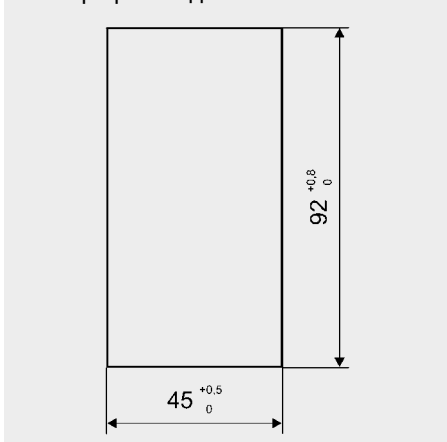
Размер проема для монтажа
